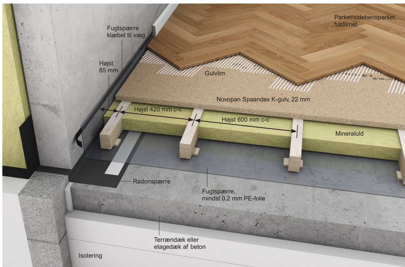
Figur 1 Novopan Spaandex K-gulv anvendt som undergulve på strøer i boliger, som underlag for fuldlimet parket og sildebensparket. På terrændæk skal strøgulvet altid udføres med en fugtspærre, der lægges direkte på betonen. Fugtspærre anbefales også på nye etagedæk og på ældre etagedæk med nyt afretningslag.
